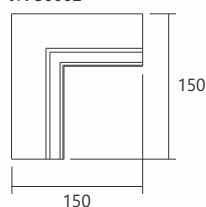
Junção Parede/Teto JN 30062
