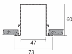
Junção Teto/Teto JN 30061
